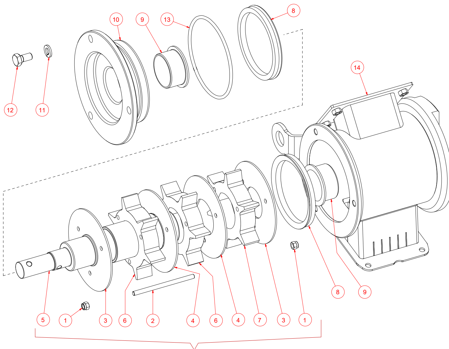
GRUPPO ROTORE COMPLETO ROTOR COMPLETE
